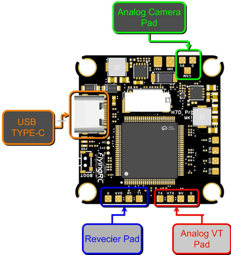
Lötpads und USB-Anschluss
