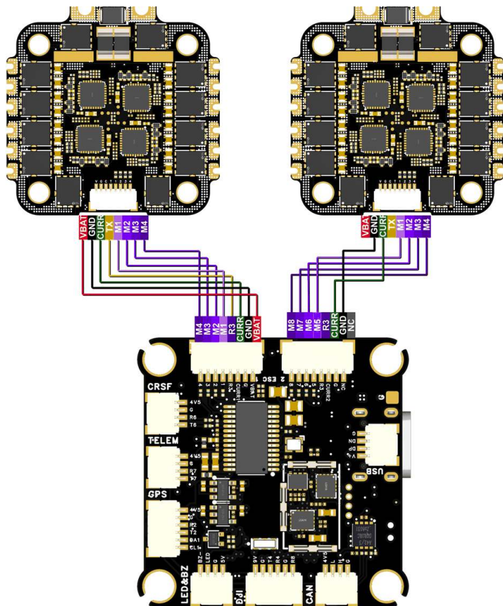
Anschluss der Flugsteuerung an die Regler nach Unterlagen des Herstellers
