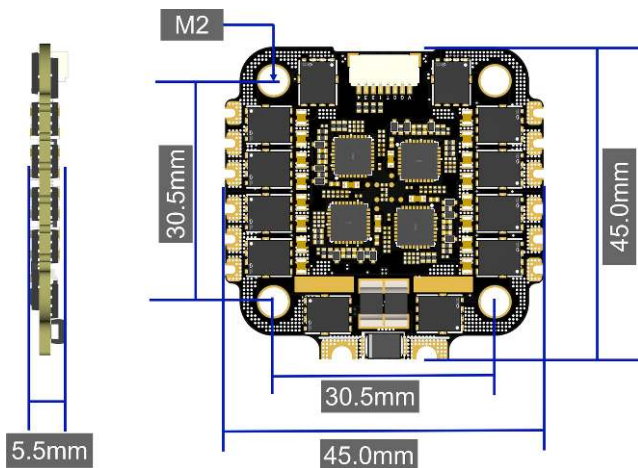
Abmessungen des Reglers
