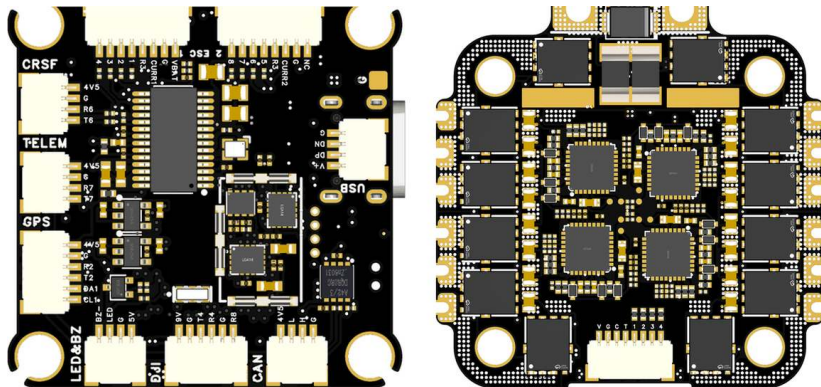
Flugsteuerung H7D Pro MK1 und 4-in-1-Regler 45 A
