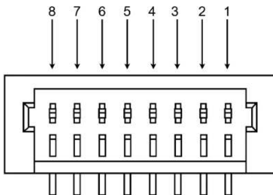
Pin-Nummerierung des SH1.0-8P-Anschlusses
